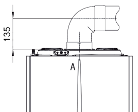
Doppelrohr-System horizontal Ø 60/100
