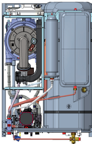
Schnittbild Victrix Zeus Superior 30
