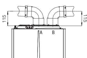
Zweirohr-System Ø 80/80
