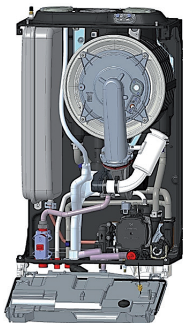
Schnittbild Victrix EXTRA 28
